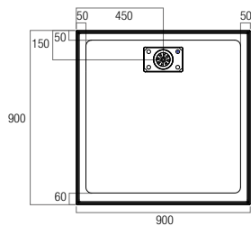
MT900R
